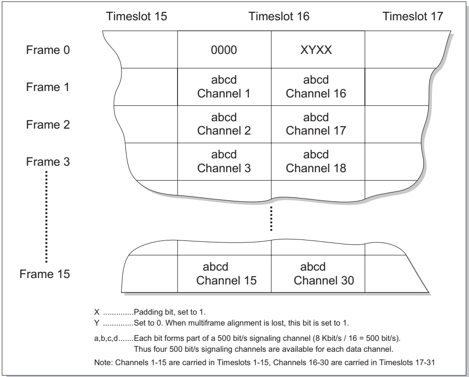
Figure 14.7 E1 Timeslot 16
