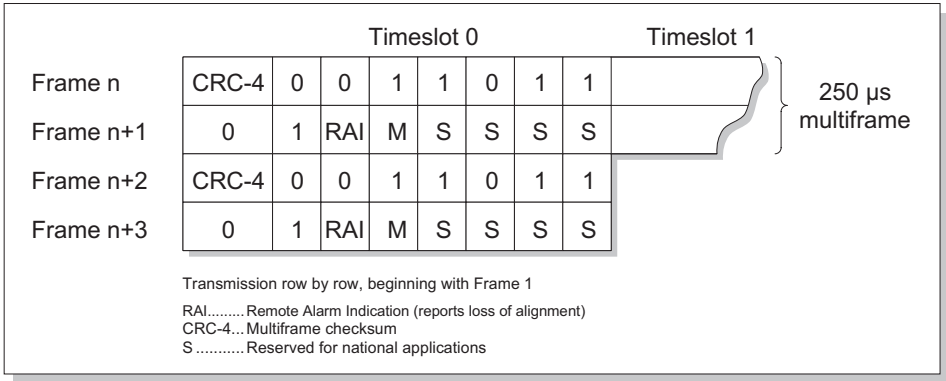
Figure 14.6 E1 Timeslot 0
